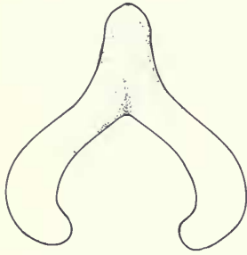
Patagona gigas
